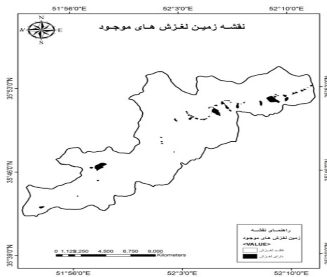
شکل (۳) پراکنش زمین لغزش های موجود در منطقه
