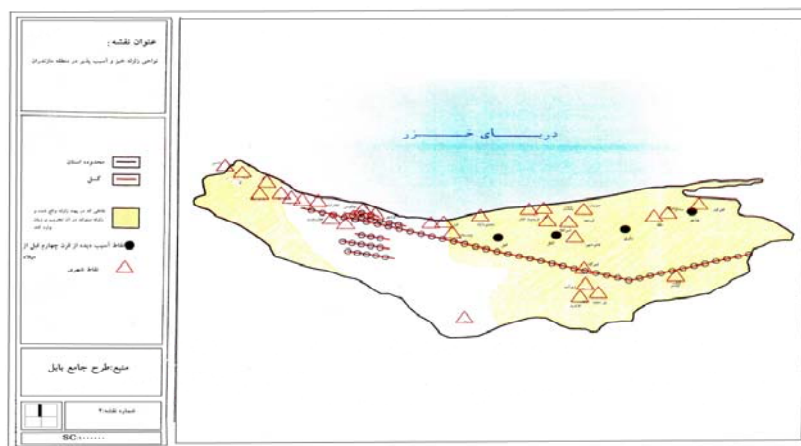
شکل (۴) نقشه پراکنده خطوط گسل در استان مازندران
