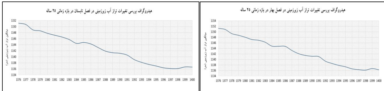
شکل (۱۵). هیدروگراف بررسی تغییرات تراز آب زیرزمینی در فصل بهار در بازه زمانی ۲۵ ساله (۱۳۷۶ - ۱۴۰۰)
