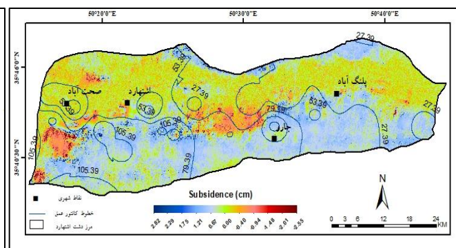
شکل (۳۴). هم پوشانی نقشه فرونشست (۲۰۲۱ - ۲۰۲۲) با میانگین تراز عمق آب زیرزمینی (۲۰۲۱)
