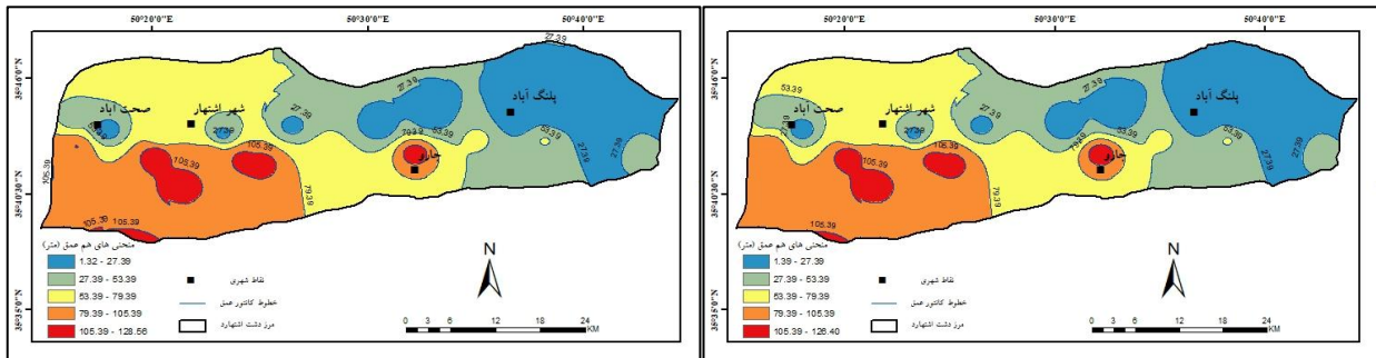
شکل (۲۴). نقشه عمق آب زیرزمینی دشت اشتهار (۲۰۱۸)
