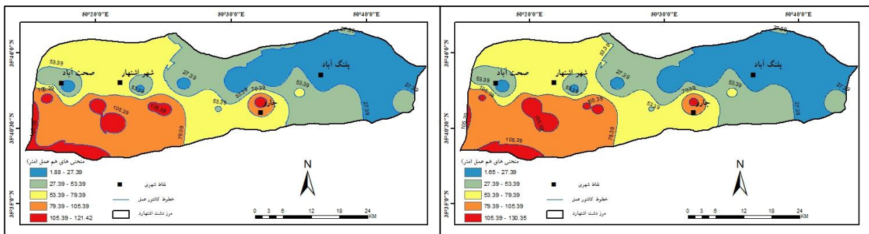
شکل (۲۷). نقشه عمق آب زیرزمینی دشت اشتهار (۲۰۲۱)
