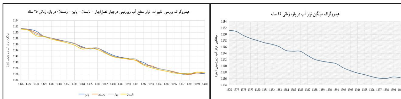
شکل (۱۹). هیدروگراف میانگین تغییرات تراز آب زیرزمینی در بازه زمانی ۲۵ ساله (۱۳۷۶ - ۱۴۰۰)
