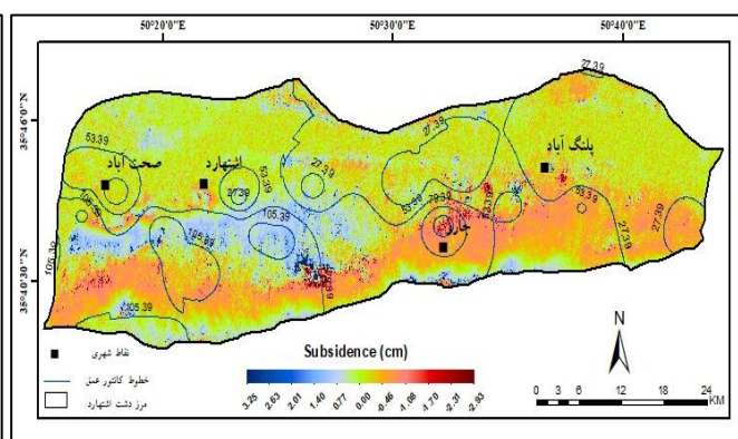
شکل (۳۲). هم پوشانی نقشه فرونشست (۲۰۱۹ - ۲۰۲۰) با میانگین تراز عمق آب زیرزمینی (۲۰۱۹)
