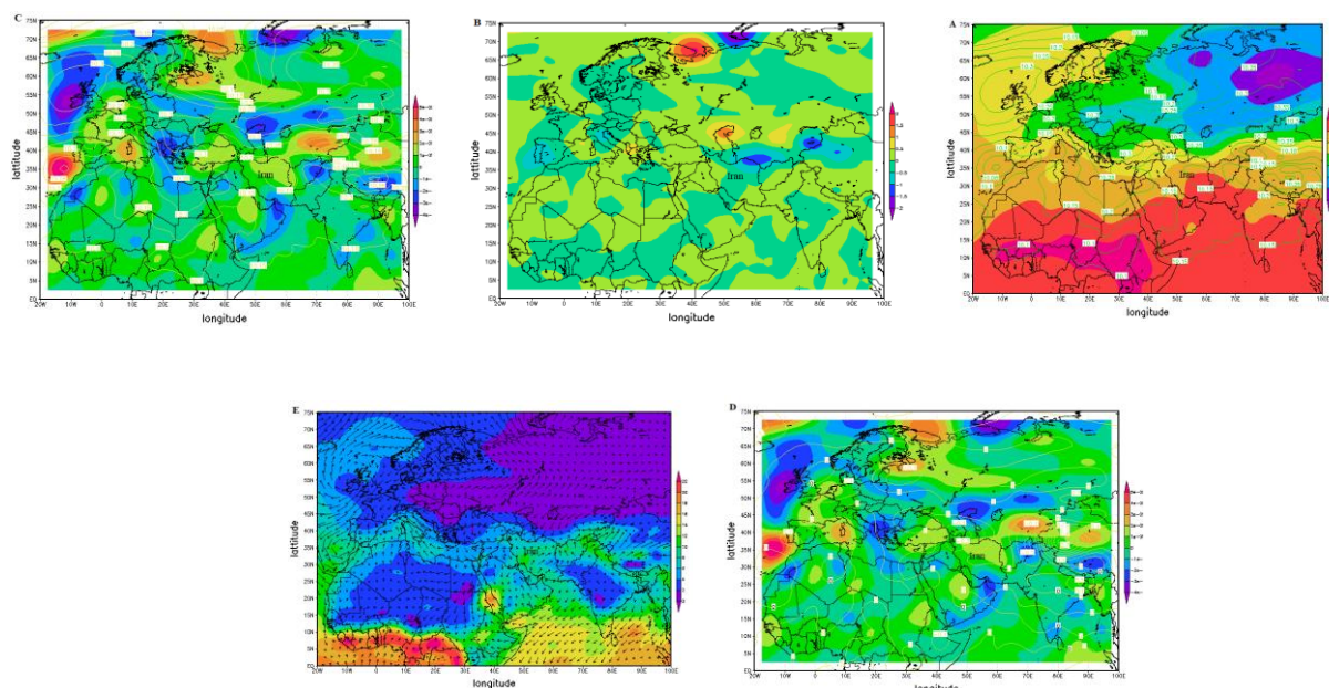
شکل (۴). روز ۲۰۰۶/۱/۲۷: (A): دما (سلسیوس، °C) و فشار (هکتوپاسکال، hPa) تراز دریا؛ (B): جبهه (کلوبین بر متر بر ثانیه و ^{\circ}F \times ms^{-1} تراز دریا؛ (C): تاوایی (متر بر ثانیه ms^{-1} ) و فشار تراز دریا (هکتوپاسکال، hPa)؛ (D): تاوایی (متر بر ثانیه ms^{-1} ) و امگا (پاسکال بر ثانیه Pa s^{-1} ) تراز دریا؛ (E): باد مداری و نصف‌النهاری و شار همگرایی رطوبت (گرم بر کیلوگرم g/kg ) تراز دریا.
