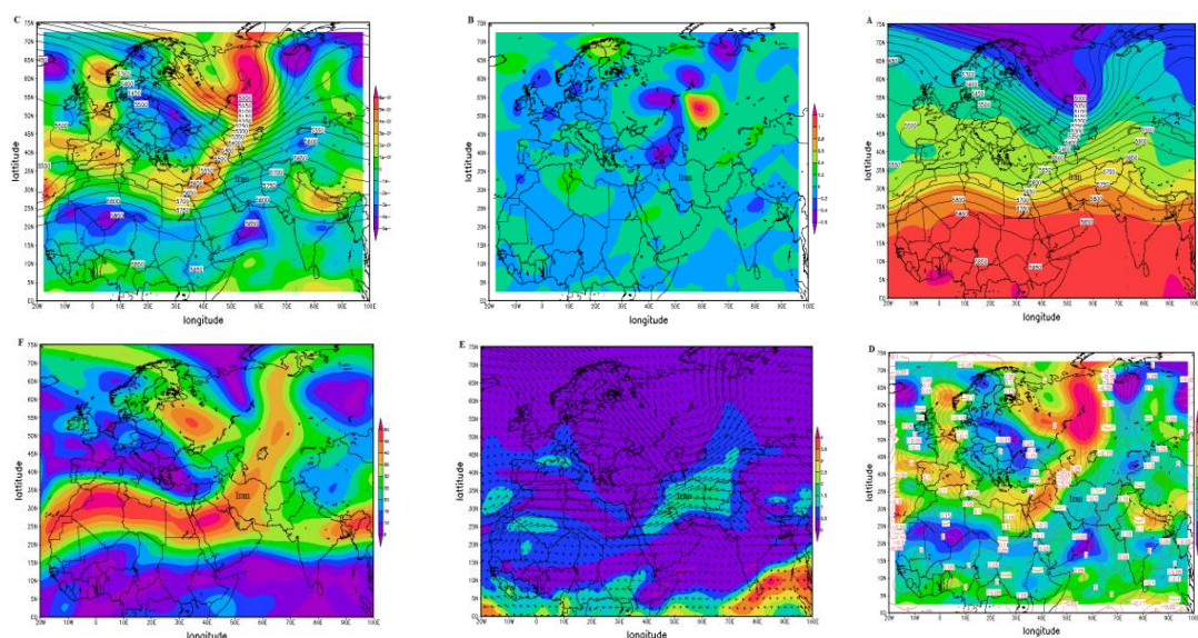
شکل (۷). (۱۹۹۶/۲/۲ A): دما (سلسیوس، °C) و ارتفاع تراز ۵۰۰ (ژئوپتانسیل متر): (B): جبهه (کلین بر متر بر ثانیه ^{\circ}F \times ms^{-1} ) (C): تاوایی (متر بر ثانیه ms^{-1} ) و ارتفاع (ژئوپتانسیل متر) تراز ۵۰۰: (D): تاوایی (متر بر ثانیه ms^{-1} ) و امگا (پاسکال بر ثانیه Pa s^{-1} ) تراز ۵۰۰ هکتوپاسکال (E): باد مداری و نصف النهاری و شار همگرایی رطوبت (گرم بر کیلوگرم ^{\circ} / kg ) تراز ۵۰۰ هکتوپاسکال: (F): جت تراز ۳۰۰ هکتوپاسکال (متر بر ثانیه m/s ).
