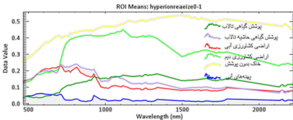
شکل (۳). متوسط بازتاب طیفی کلاس‌های انتخاب شده الف- تصویر ALI ب- تصویر ETM+ ج- تصویر Hyperion
