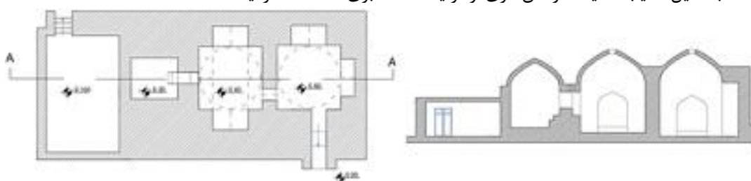
شکل (۱۳). پلان حمام خانجمال (منبع: آرشو میراث فرهنگی استان کرمانشاه، ۱۳۹۹)
