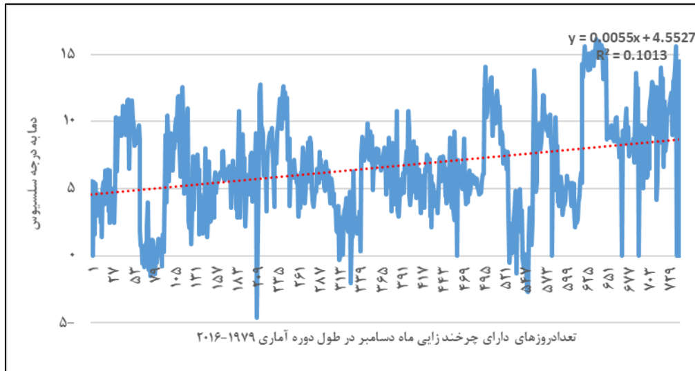
شکل (۲۶). میانگین دمای مراکز چرخندی در ماه دسامبر در طول دوره آماری ۱۹۷۹-۲۰۱۶
