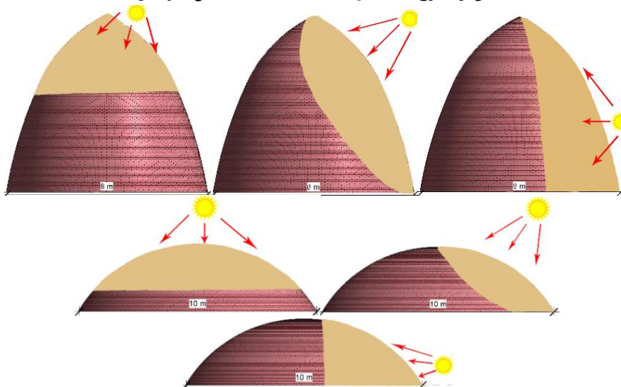
شکل (۱۰). از سمت بالا تصاویر گرافیکی میزان دریافت تابش بر سطوح گنبد خیز بلند در سه بازه‌ی زمانی روز (۱۳، ۱۴، ۱۶). از سمت پایین تصاویر گرافیکی میزان برخورد تابش خورشید بر سطوح گنبد آبنا‌های خیز کم در سه بازه‌ی زمانی روز (۱۳، ۱۴، ۱۶). منبع: نگارندگان.
