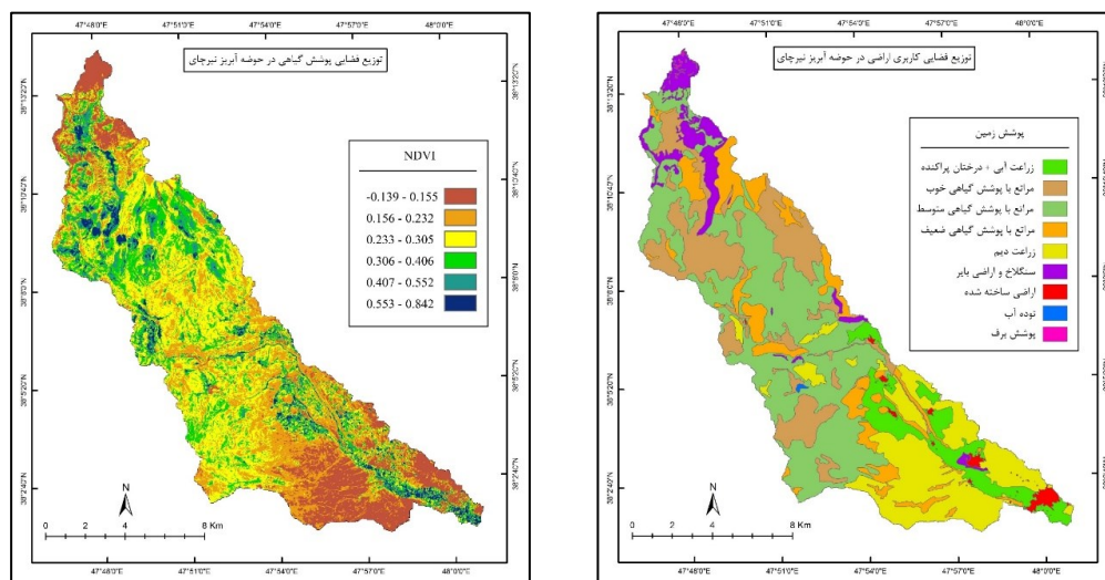
شکل (۳). نقشه کاربری اراضی حوضه نیرچای
