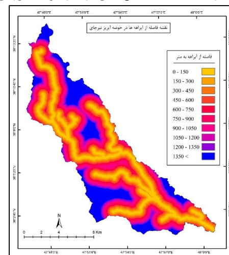
شکل (۱۹). نقشه فاصله از آبراهه‌های حوضه نیرچای
