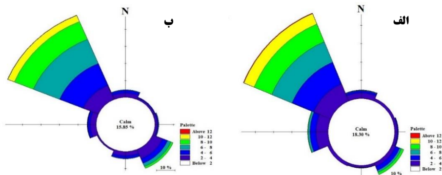
شکل (۸). گلباد نقطه‌ای واقع در مرکز خلیج فارس در (الف) فصل گرم و (ب) فصل سرد
