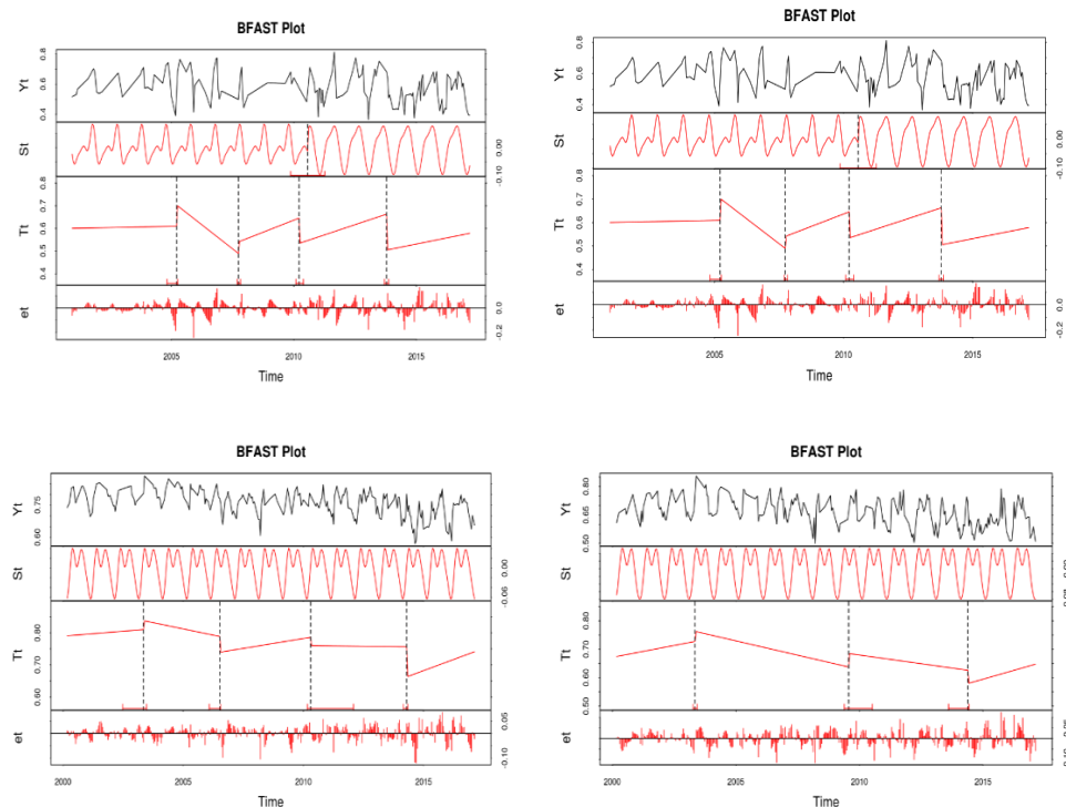
شکل (۱۱). نمودار BFAST از مناطق حائز تغییرات در جنگل‌های بلوط
