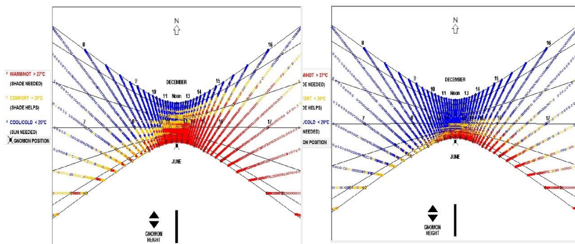
شکل (۵). حرکت سایه خورشید دوره (تابستان-پاییز)
