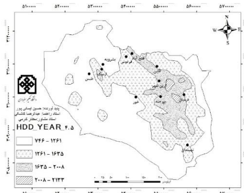
شکل (۳۲). پراکنش مکانی نیازهای گرمایشی سالانه دوره آینده (۲۰۱۶-۴۱) سناریو RCP_4.5
