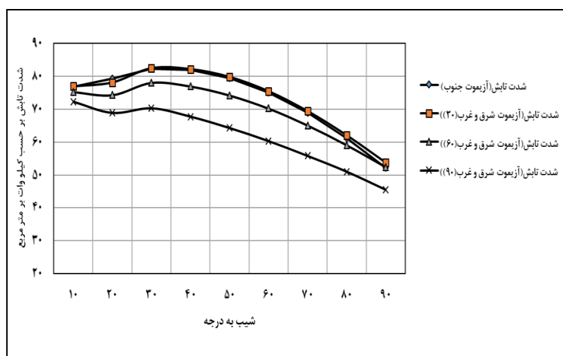
شکل (۷). مجموع تابش دریافتی روزانه در سال از خورشید بر سطح کلکتور با آزمون‌ها و زوایای شیب مختلف شهرستان کاشان (کیلو وات بر متر مربع)
