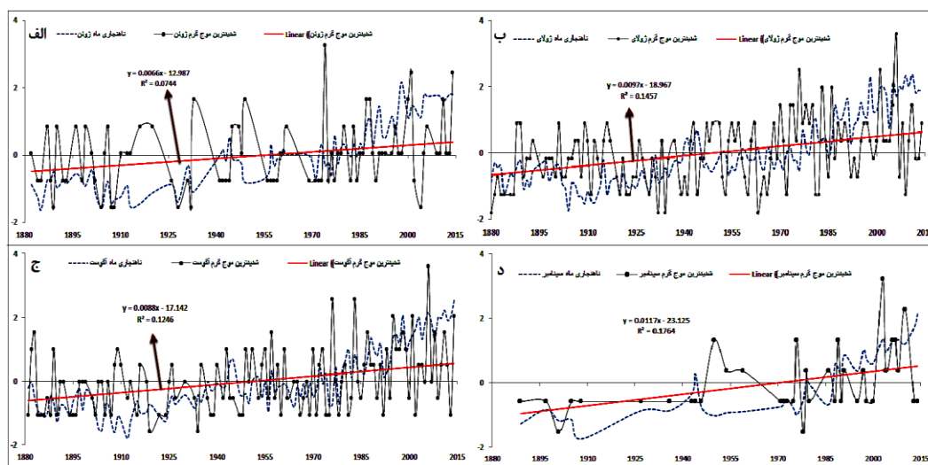
شکل (۱۰). نمودار مقایسه‌ای و استاندارد شده‌ی ماماهاهی رخداد شدیدترین امواج گرم با ناهنجاری دمایی اقیانوس و خشکی در منطقه شمال غرب ایران، الف (ژوئن)، ب (ژوئای)، ج (آگوست)، د (سپتامبر) در بازه زمانی ۱۸۸۰ تا ۲۰۱۴.
