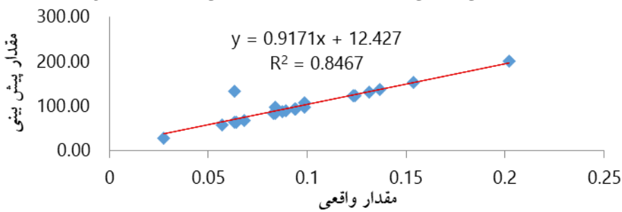
شکل (۲) رابطه همبستگی خروجی‌های الگوی دوم با داده‌های واقعی در ماه ژانویه منبع: نگارندگان
