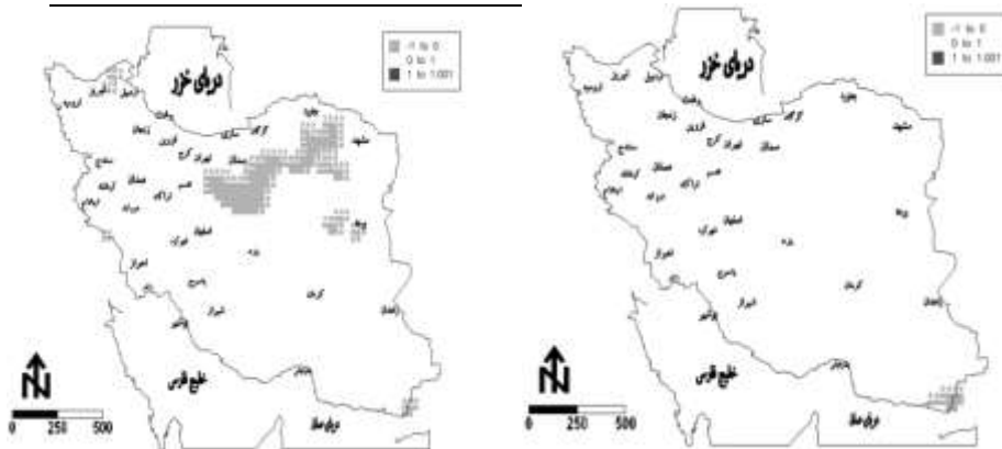
شکل (۱۱). روند دمای ماه سپتامبر در قلمرو ایران طی دوره آماری ۲۰۱۵-۲۰۵۰
