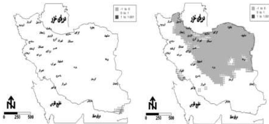
شکل (۱۳). روند دمای ماه نوامبر در قلمرو ایران طی دوره آماری ۲۰۱۵-۲۰۵۰
