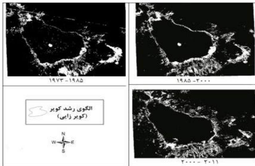
شکل (۵) تغییرات و گسترش مساحت کویر طی دوره های زمانی ۱۹۷۳-۲۰۱۱
