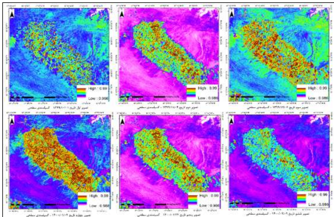
شکل (۴). نتایج حاصل از گسیلمندی سطحی
