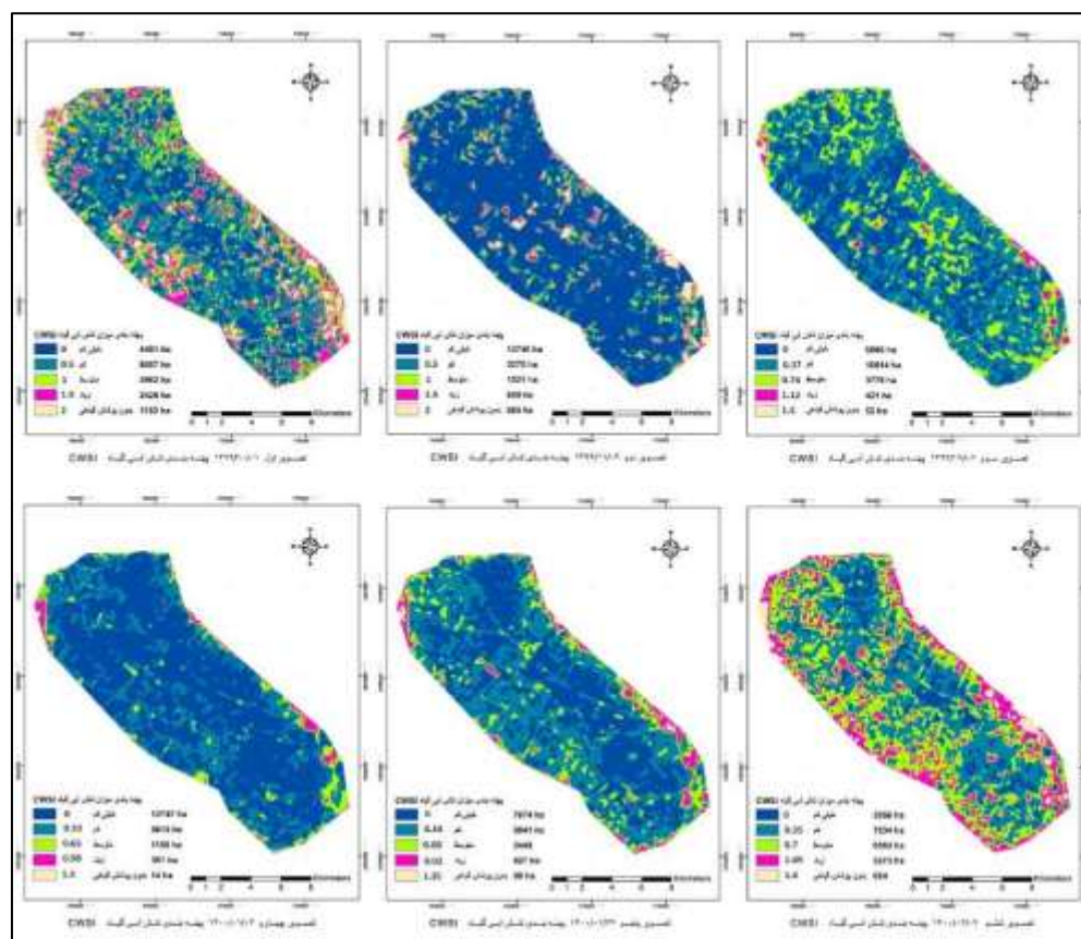
شکل (۸). پهنه‌بندی تنش آبی گیاه (CWSI)
