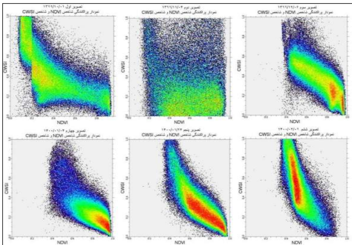
شکل (۱۰). نمودار پراکندگی NDVI و شاخص CWSI
