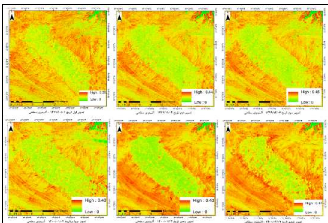
شکل (۲). مقدار آلبیدوی سطحی به دست آمده از تصاویر لندست-۸
