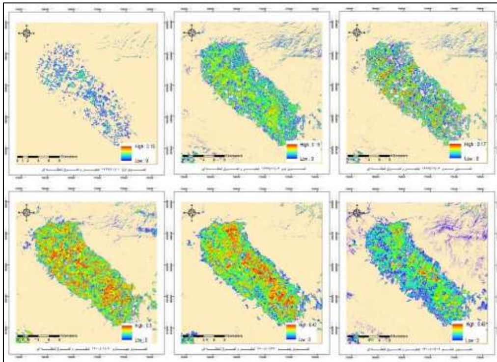
شکل (۶). کسر تبخیر-تعرق مرجع (میلی‌متر در ساعت)
