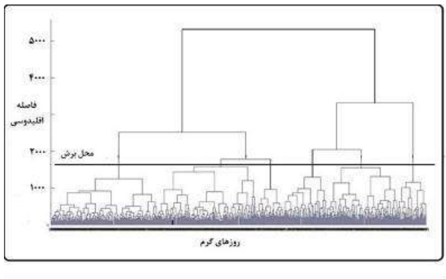
شکل (۲). دارنمای داده‌های فشار تراز دریا مربوط به روزهای گرم فرین فراگیر + منبع: نگارنده
