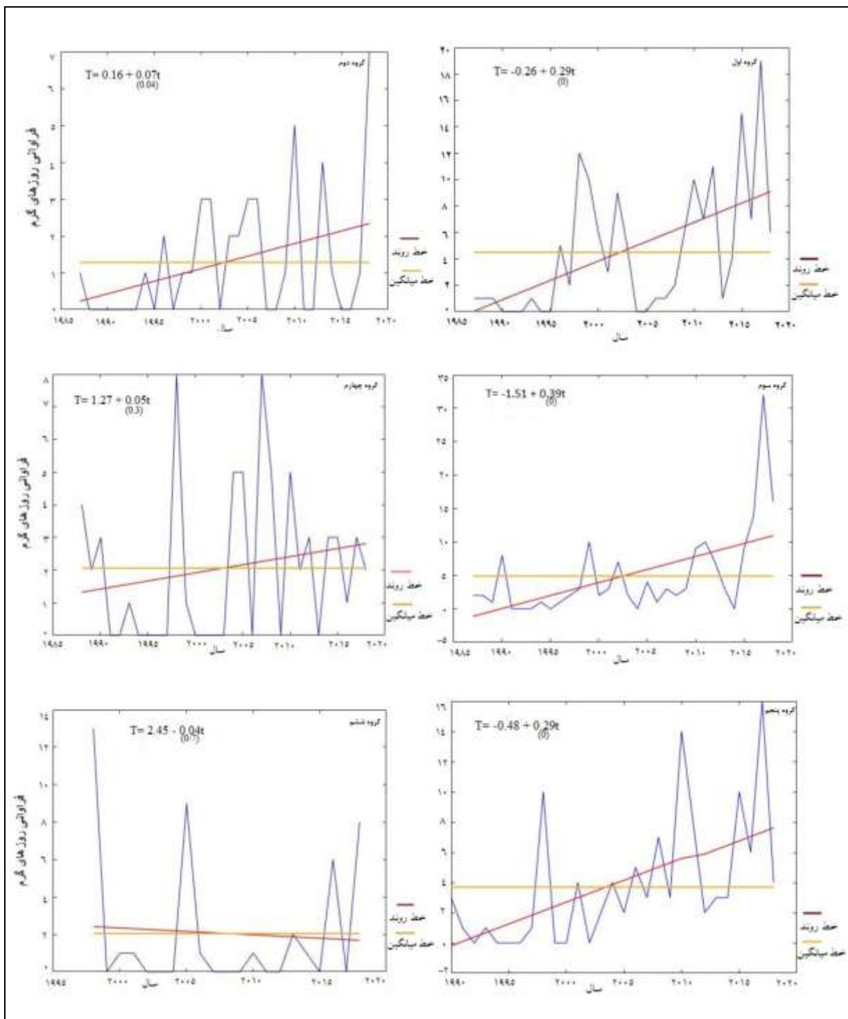
شکل (۴). فراوانی سالانه روزهای گرم فراگیر و روند آن‌ها برای گروه اول تا گروه ششم منبع: نگارنده
