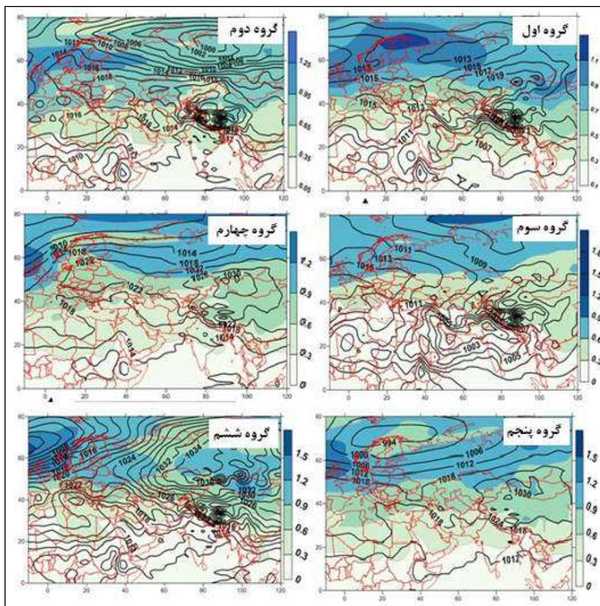
شکل (۳). میانگین فشار تراز دریا (هم‌مقدارها به هکتوپاسکال) و ضریب تغییرات (پس‌زمینه رنگی به درصد) برای گروه اول تا گروه ششم منبع: نگارنده
