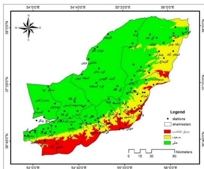
شکل (۳). پهنه‌بندی مناطق مستعد کشت چغندر قند پاییزه در مراحل مختلف فنولوژیکی (جوانه زدن، هشت برگ، حجیم شدن ریشه و تجمع قند و رسیدن کامل) از نظر دمای در استان گلستان منبع: نگارندگان، سال ۱۴۰۱
