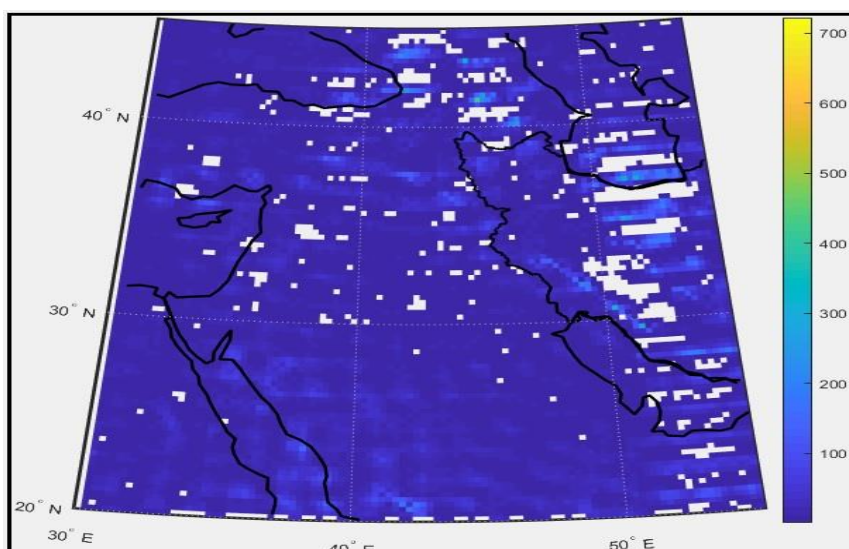
شکل (۱۵). مکان چرخندزایی و گذر چرخندی در ماه مارس در طول سال‌های آماری ۲۰۱۶-۱۹۷۹، (آبی پررنگ چرخندزایی ضعیف و طیف رنگی متمایل به زرد چرخندزایی، مربع‌های سفید نشانه عدم رخ داد چرخندزایی)
