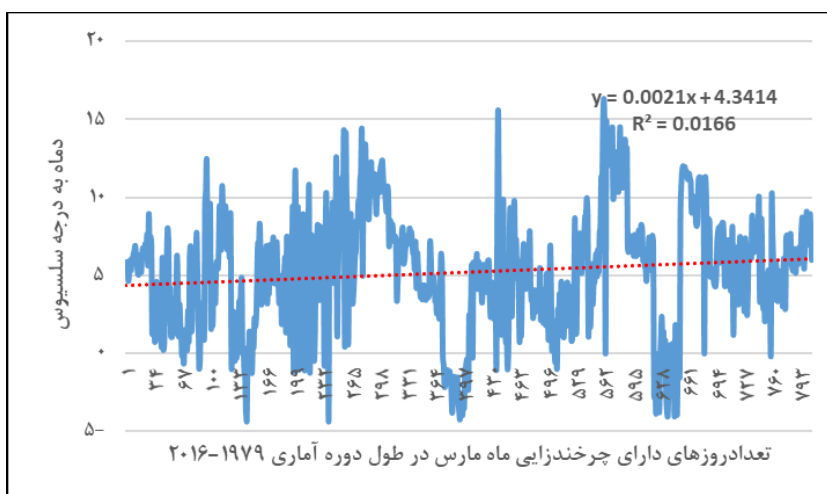
شکل (۱۴). میانگین دمای مراکز چرخندی در ماه مارس در طول دوره آماری ۲۰۱۶-۱۹۷۹
