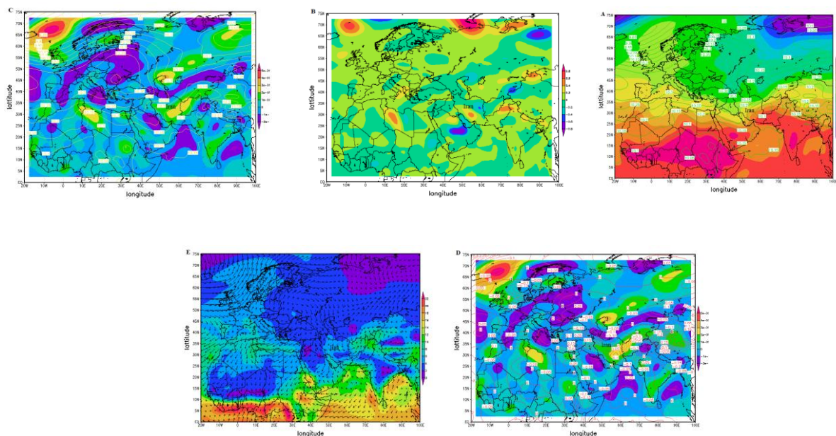
شکل (۸). ۱۹۹۲/۳/۱۰: (A): دما (سلسیوس، °C) و فشار (هکتوپاسکال، hpa) تراز دریا؛ (B): جبهه تراز دریا (کلون بر متر بر ثانیه ^{\circ}\text{F} \times \text{ms}^{-1} )؛ (C): تاوایی (متر بر ثانیه \text{ms}^{-1} ) و فشار تراز دریا (هکتوپاسکال، hpa) (D): تاوایی (متر بر ثانیه \text{ms}^{-1} ) و امگا (پاسکال بر ثانیه \text{Pa s}^{-1} ) تراز دریا (E): باد مداری و نصف‌النهاری و شار همگرایی رطوبت (گرم بر کیلوگرم \text{g/kg} ) تراز دریا.
