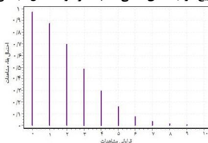
ج: نمودار تابع احتمال بقاء توزیع دو جمله‌ای منفی
