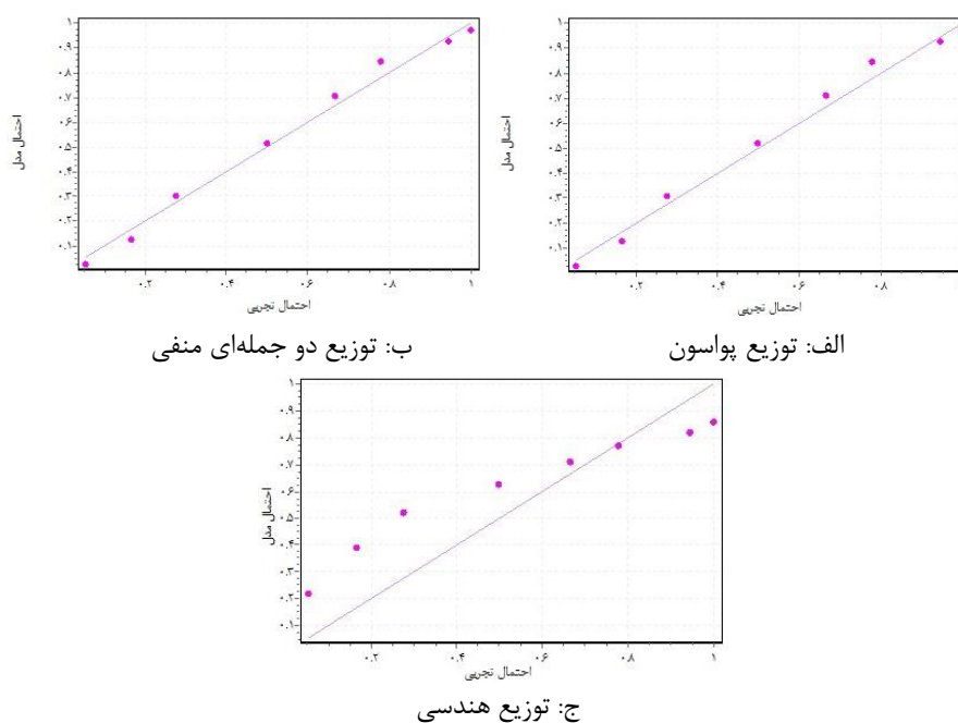
شکل (۲). نمودار احتمال - احتمال (p-p) برای مشاهدات جدول ۴ ایستگاه بانه (۲۰۱۴-۱۹۹۲)
