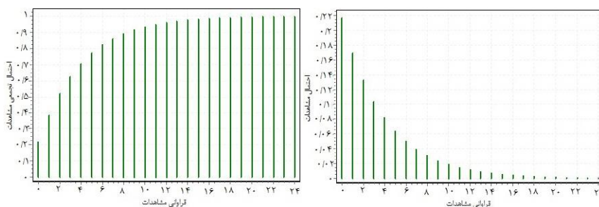
الف: نمودار تابع احتمال توزیع هندسی ب: نمودار احتمال تجمعی توزیع هندسی
