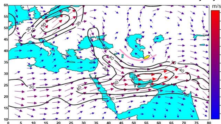
شکل (۹). میدان باد تراز ۳۰۰ هکتوپاسکال (متر بر ثانیه) در ساعت ۰۰۰۰ گرینویچ روز ۱۸ مارس ۲۰۱۹
