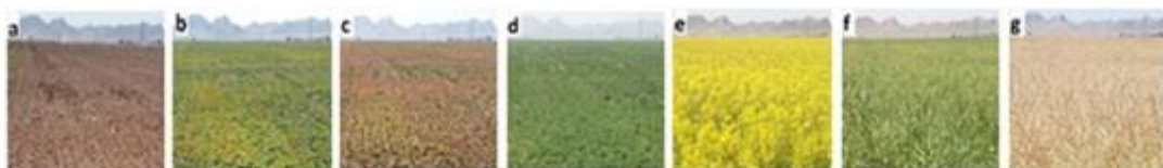
شکل (۲). مراحل فنولوژی گیاه کلزا: (a) - (کاشت) - (b) - (رزت) - (c) - (رکود) - (d) - (رویش مجدد) - (e) - (گلدهی) - (تشکیل غلاف) - (f) - (رسیدن) - (g)
