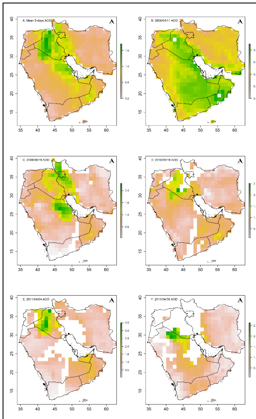
شکل (۱۰). پراکنش مکانی عمق نوری آتروسل (MODIS (AOD 550nm بر روی خاورمیانه، A: میانگین ۵-روزه فرین‌های گردوغبار، B: فرین ۲۰۰۸/۰۴/۱۱: C: ۲۰۰۹/۰۶/۱۹: D: ۲۰۱۰/۰۵/۱۹: E: ۲۰۱۱/۰۴/۰۴ و F: ۲۰۱۱/۰۴/۳۰-روزه
