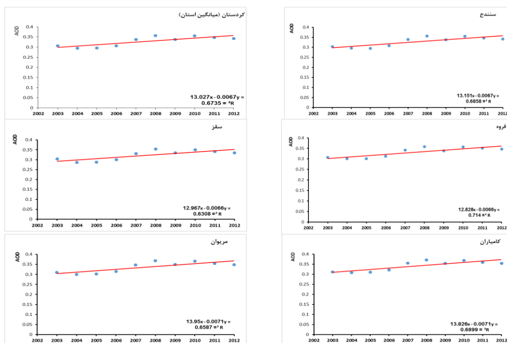
شکل (۱). میانگین سالانه عمق نوری آئروسول (AOD 550nm) در استان کردستان (۲۰۱۲-۲۰۰۳)
