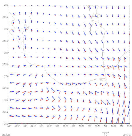
شکل (۶). نقشه ماهانه بردار باد سطح زمین در ساعت ۰۰ GMT، شرایط مرجع (خطوط آبی) و شرایط حاصل از حذف توپوگرافی (خطوط قرمز)
