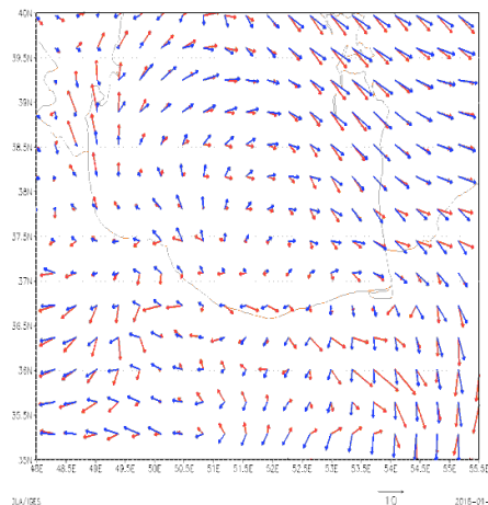
شکل (۱۰). نقشه بردار باد سطح زمین در ساعت GMT ۱۲ روز ۲۷ جولای ۲۰۰۲، شرایط مرجع (خطوط قرمز) و شرایط حاصل از حذف توپوگرافی (خطوط آبی)
