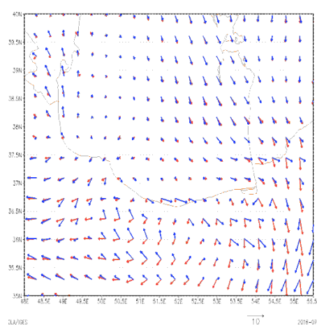
شکل (۵). نقشه ماهانه بردار باد سطح زمین در ساعت ۱۲ GMT، شرایط مرجع (خطوط آبی) و شرایط حاصل از حذف توپوگرافی (خطوط قرمز)
