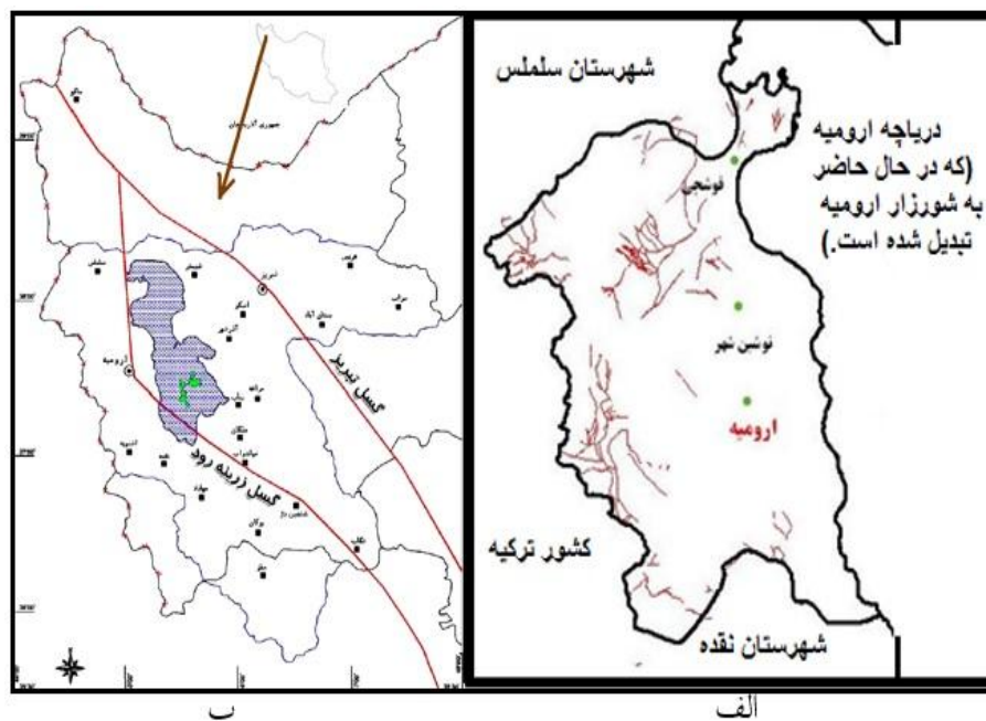
شکل (۲). الف) شبکه سیستم های گسلی و شکستگی های منطقه مورد مطالعه (اقتباس از نقشه زمین شناسی ۱:۱۰۰۰۰۰ منطقه). و ب) گسل های اصلی و بزرگ ارومیه و تبریز (آقاباتی ۱۳۸۳ ص ۶۴۴).
