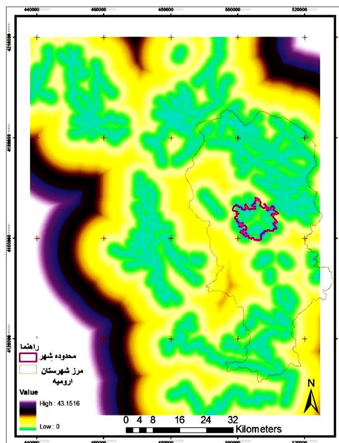
شکل (۵). لایه فاصله از شکستگی های زمین (اقتباس از آمبرسیز ۱۹۸۸)
