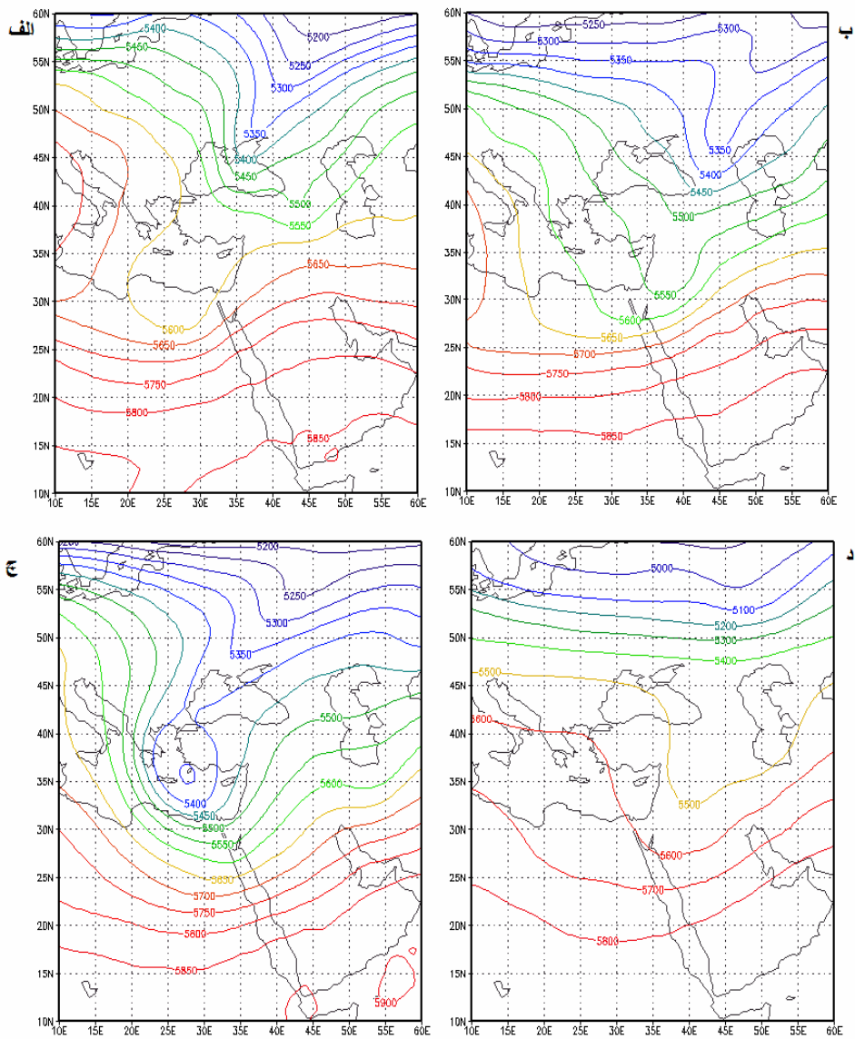
شکل (۱) مکان گزینی ناوه سامانه ترکیبی مدیترانه‌ای- سودانی در ساعات مختلف تراز ۵۰۰ هکتوپاسکال، (الف) ساعت 00 روز 4 فوریه ۱۹۹۵ (ب) ساعت ۱۸ utc روز ۴ فوریه ۱۹۹۵ (ج) ساعت ۱۸ utc روز ۶ فوریه ۱۹۹۵ (ب) ساعت ۱۸ utc روز ۸ فوریه ۱۹۹۵
