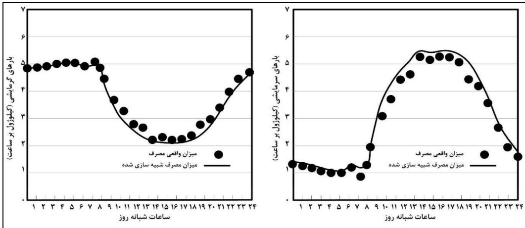
شکل (۲). مقایسه نتایج مصرف انرژی سرمایه‌ی و گرمایشی حاصل از شبیه‌سازی و میزان واقعی مصرف برای یک دوره ۲۴ ساعته.
