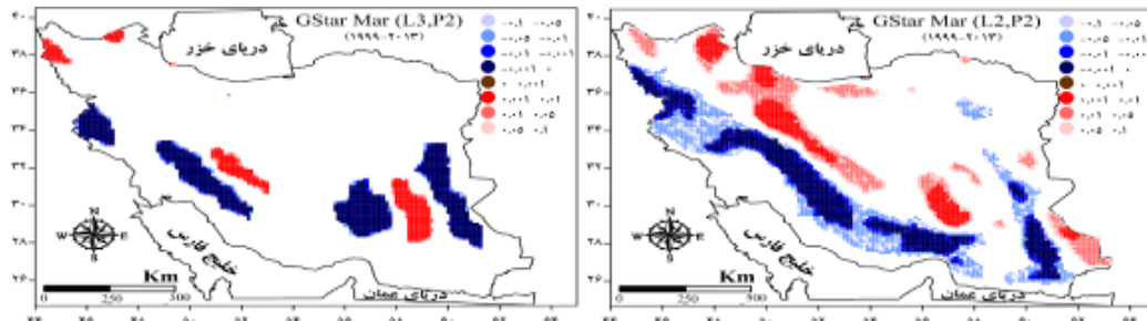
شکل (۳). نقشه‌های خودهمبستگی فضایی VIMFC ژانویه تا مارس بر روی ایران طی دوره اول ۱۹۷۹-۱۹۹۸ (P1) و دوم ۱۹۹۹-۲۰۱۳ (P2). منظور از L1 لایه اول، L2 لایه دوم، L3 لایه سوم است.
