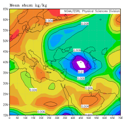
شکل (۵) نقشه میانگین تراز ۵۰۰ هکتوپاسکال در الگوی دوم
