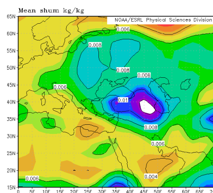
شکل (۶) نقشه رطوبت ویژه روز نمونه الگوی دوم در تراز ۸۵۰ هکتوپاسکال (۲۴ ژوئن ۱۹۸۱)
