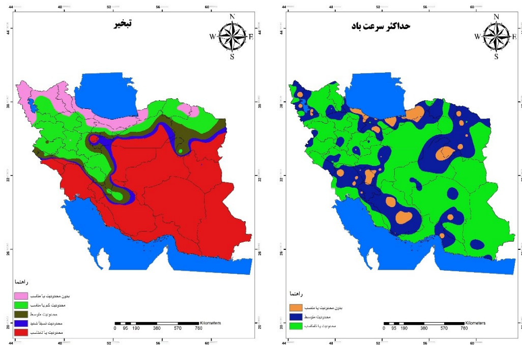
شکل (۱۱). نقشه تبخیر و تعرق
