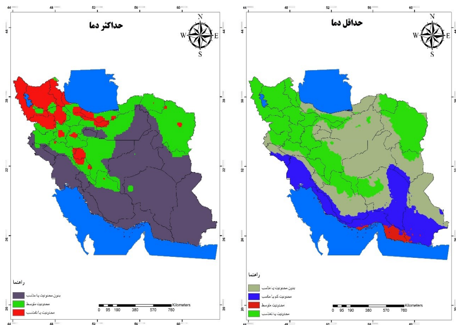
شکل (۱۳). نقشه حداکثر دما
