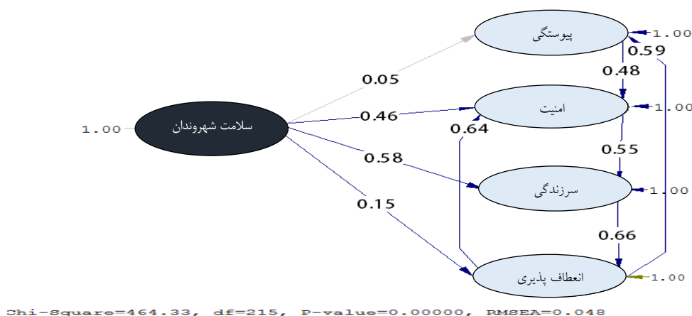
شکل (۵). مدل ساختاری (SEM) ضریب پیوستگی پیرسون و ارتباط بین ساماندهی رود دره و شاخص سلامت شهر وندان
