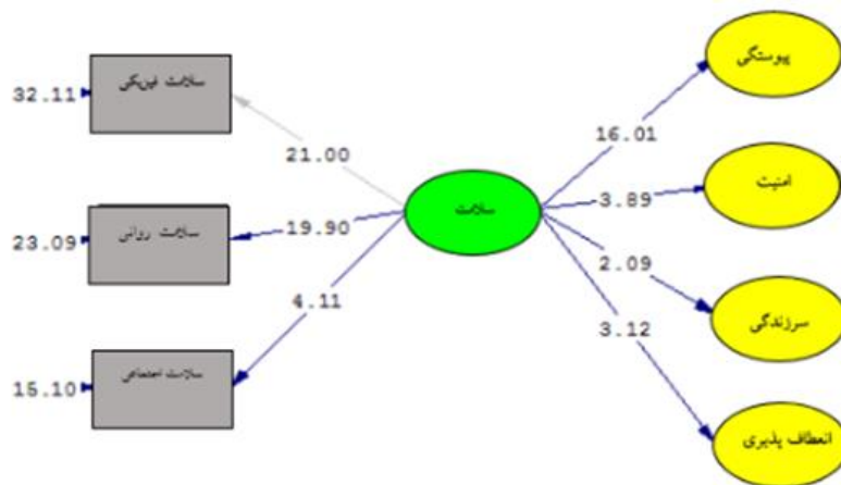
شکل (۶). مدل ساختاری (sem) تحقیق جهت نمایش درستی ارتباط میان تأثیر ساماندهی رود دره بر سلامت شهروندان بر اساس آماره T
