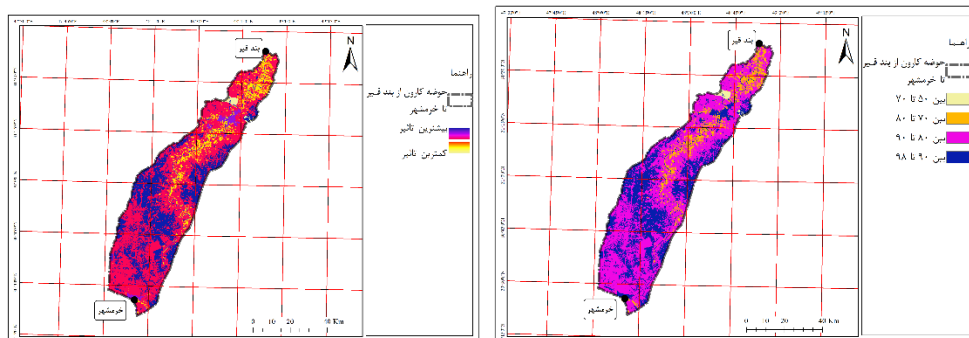
نقشه نفوذپذیری خاک (CN) حوضه نرمال شده
