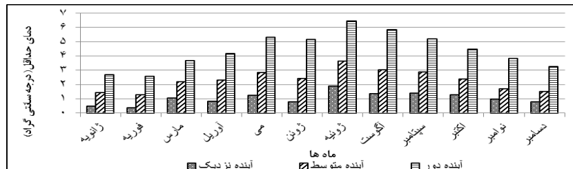
شکل (۸). تغییرات میانگین دمای حداقل ماهانه دوره مشاهداتی و آینده ایستگاه آرازکوسه
