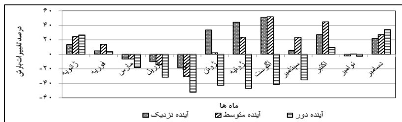
شکل (۷). درصد تغییرات میانگین بارش ماهانه دوره مشاهداتی و آینده ایستگاه آرازکوسه
