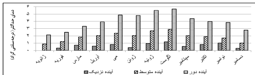
شکل (۹). تغییرات میانگین دمای حداکثر ماهانه دوره مشاهداتی و آینده ایستگاه آرازکوسه
