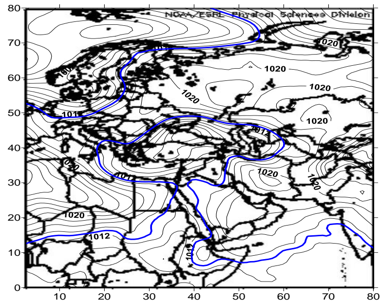
شکل (۶). نقشه الگوی تراف عمیق (الف: سطح ۵۰۰) و (ب: فشار سطح دریاها) آزاد
