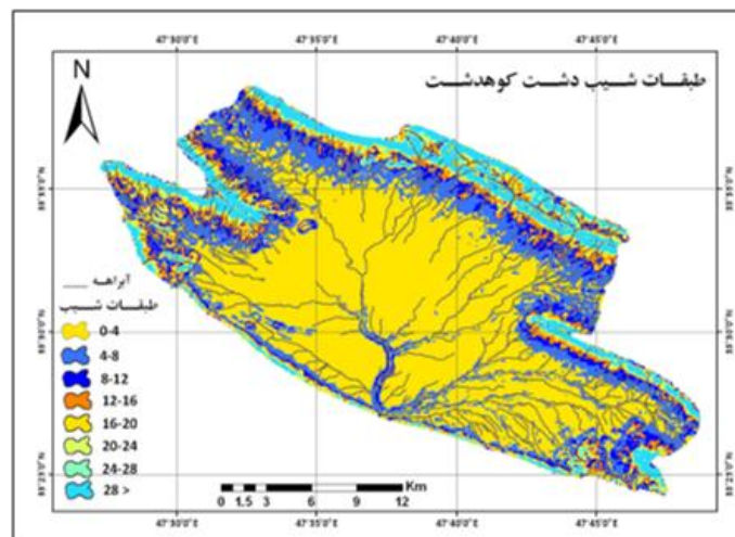
شکل (۱۳) شیب طبقاتی دشت کوهدشت
