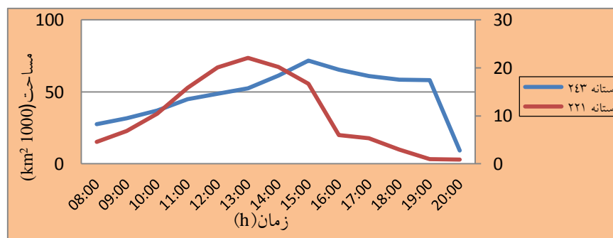
شکل (۲). مقایسه تغییرات مساحت سامانه‌های همرفتی میان‌مقیاس در دو آستانه ۲۲۱ و ۲۴۳ کلوین
